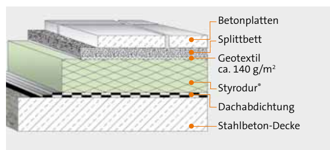
Abb. 69: Aufbau eines UK-Terrassendaches mit Betonplatten im Splittbett.
