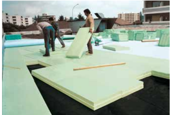
Abb. 43: Verlegung von Styrodur® beim Duodach.
