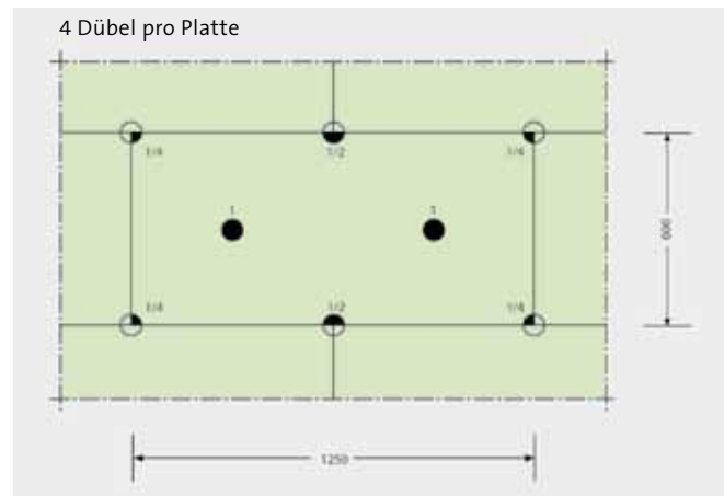
Abb. 24: Dübelanzahl (4 Dübel pro Platte) und Dübelanordnung bei nachträglicher Befestigung von Styrodur® C-Platten im Sockelbereich (Maße in mm).
