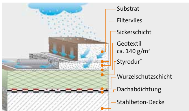
Abb. 60: Schichtenaufbau eines begrünten Umkehrdaches mit Dränschicht zur flächigen Wasseraufnahme und alternativ mit Dränleitung.
