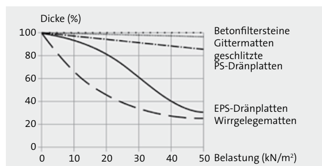
Abb. 61: Zeitstandverhalten verschiedener Dränelemente nach 50 Jahren. Dickenänderung in Abhängigkeit von der Belastung.
