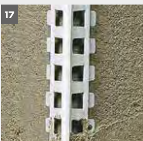
WDVS mit Hochleistungs-Dämmplatten aus Resol-Hartschaum und dickschichtigem Putzaufbau
