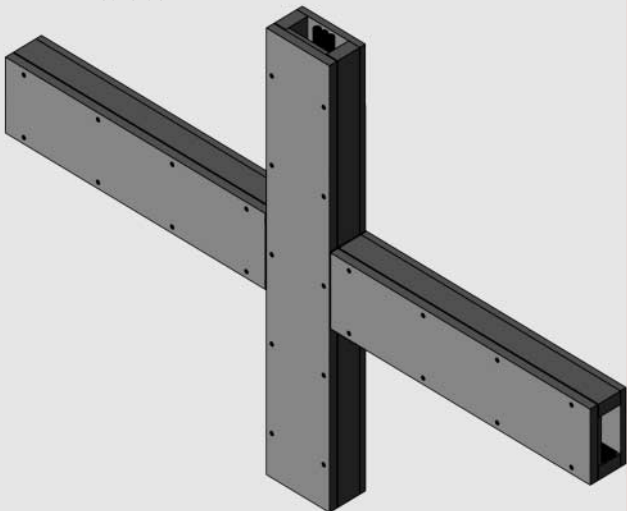
Kreuzstück
