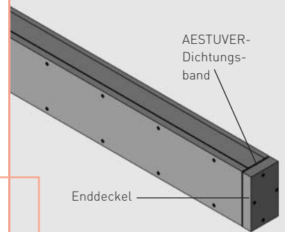
Endstück
